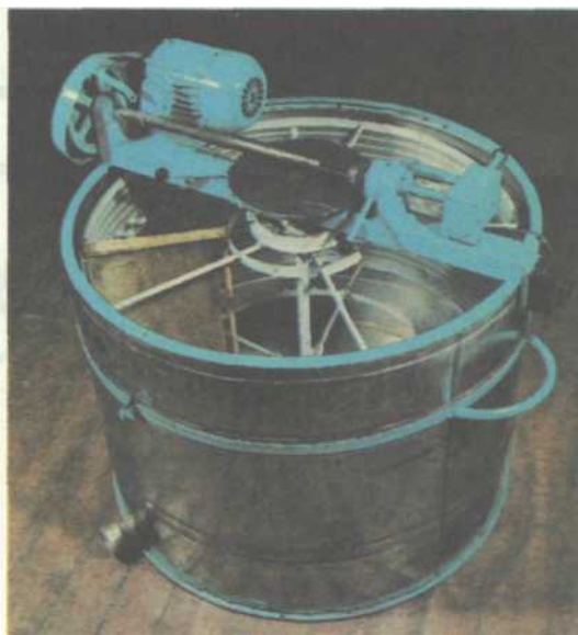
Рис. 72. Медогонка радиальная электрифицированная на 50 рамок.
