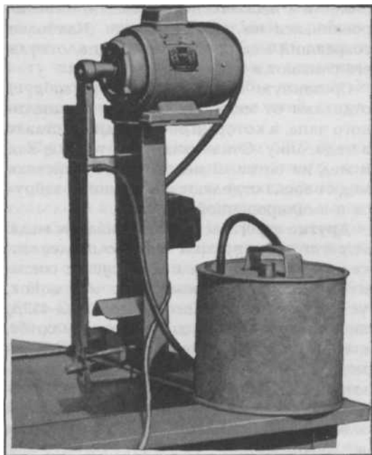
Рис. 35. Вибронож.
