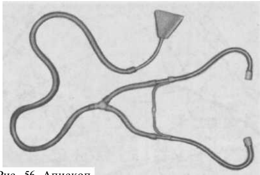
Рис. 56. Апископ.
